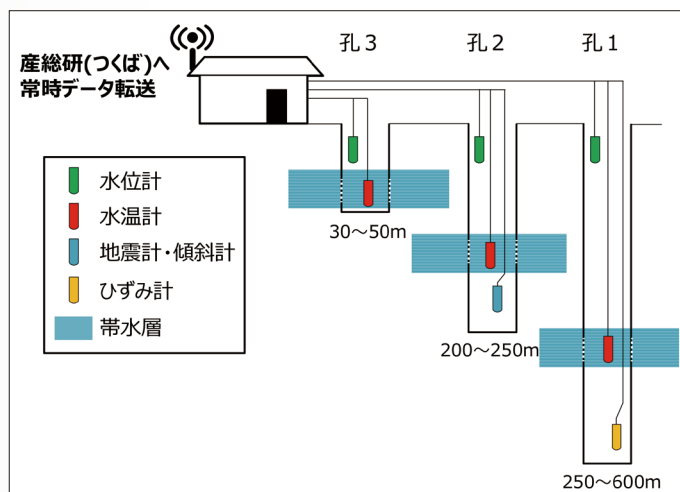
図2 ひずみ・地下水等観測施設の概要 地上に観測建屋があり、3本の観測井戸の中に計測機器類を設置しています。
