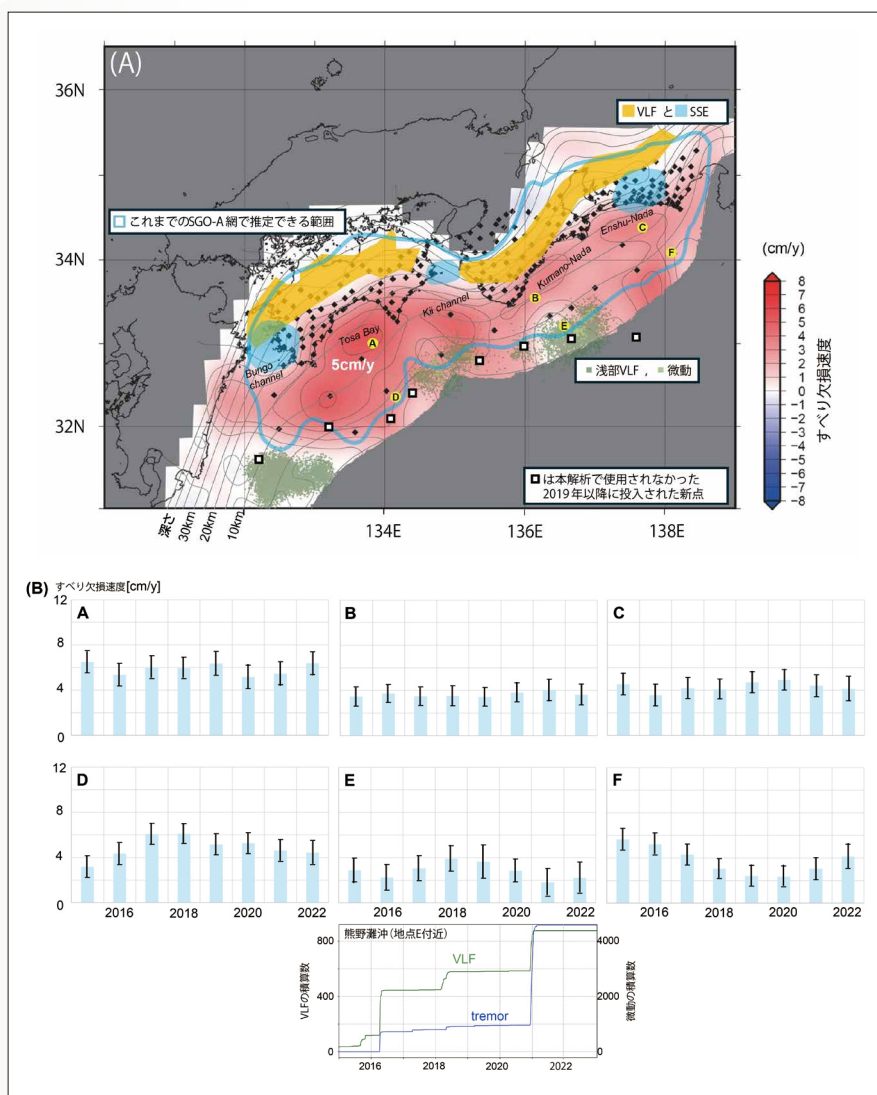
図1 (A) 本研究で推定したすべり欠損速度の全期間の最小値の分布。すべり欠損速度は固着状態の指標となり、赤色の濃い領域が長期にわたって固着が強い範囲を示す。黄色および水色の領域は、深部低周波微動活動域および2013年以降の深部スロースリップの分布域である。緑色の点は浅部VLFと微動の分布、水色の線はこの解析が解能を有する範囲を示す。 (B) Aの各地点におけるすべり欠損速度の時間変化。棒グラフは、各時間窓における推定値 \pm 1\sigma （左縦軸）を示している。下段は2014年以降のVLFおよび微動の積算数。※図中の引用については参考文献をご参照ください 7 。
