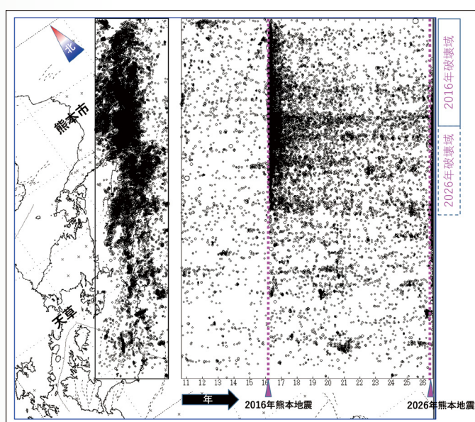
図2 2016年熊本地震前後の地震活動。左図は地震が発生した場所を地図上に示したもの。右図は、左図の黒枠内で発生した地震について、横軸を時間として示したもの。「2016年破壊域」は、2016年熊本地震で断層が大きくずれた範囲を示す。また「2026年破壊域」は震源分布から予想した暫定的なものを示す。
