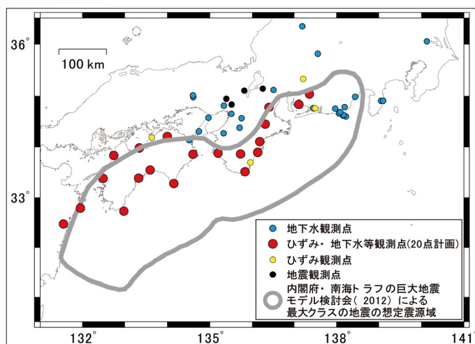
図1 産総研のひずみ・地下水等観測網 水色と黄色の丸：20点計画以外の地下水観測点とひずみ観測点
