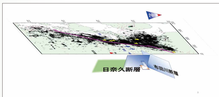
図1 余震の震源分布から推定した2016年熊本地震の地下の断層の形状。青とオレンジの面が2016年熊本地震の震源断層を示す。緑は2026年熊本地震の破壊域(暫定的に設定)。地表には2016年熊本地震から1年間に発生した地震の震央を示している。☆はマグニチュード5以上の地震の震央。地表断層をピンク線で示す。
