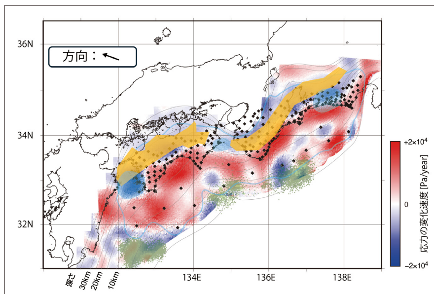
図2 図1の最小すべり欠損速度分布から算出された、N290E方向における応力変化速度の分布。赤色の濃い領域がフィリピン海プレートの沈み込みにより応力を高めている領域。領域や点の分布については図1(A)と同じ。
