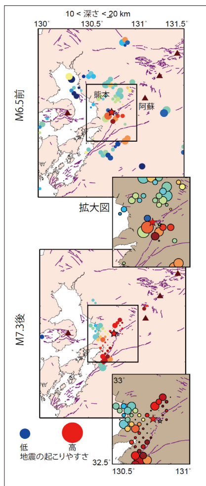
図3 深さ10kmから20kmまでのb値と地震の臨界度を組み合わせた地震活動の評価。地図の枠で囲んだ部分を拡大した分布図を右下に示す。色が青から赤になるほどb値が低く、地下の岩盤にかかる力が大きいことを示す。丸が大きいほど臨界度が高く、大きな規模の地震へ発展しやすい状態を示す。地震前には、本震の震源(★)付近でこの二つの特徴が同時に見られる。地震後には、そのような場所が周辺にも広がっている。紫の線は活断層を示す。(文献 4) を改変)
